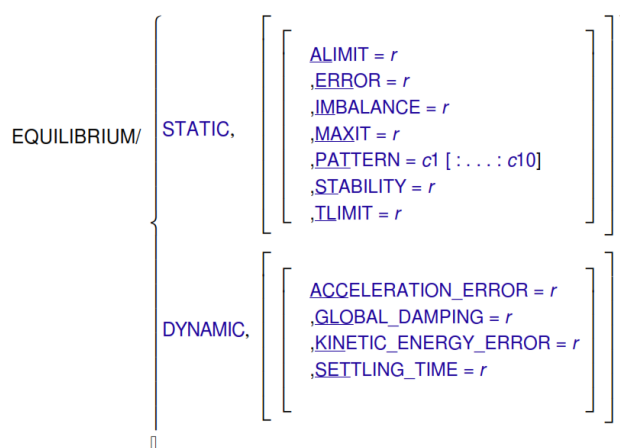
Slika 52. Struktura postavki i rubnih uvjeta Solver-a pri rješavanju simulacije, izvadak iz [19]
