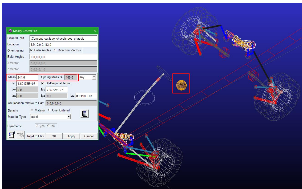
Slika 106. Definiranje ovješene mase bolida u modelu vozila u Adams CAR-u
