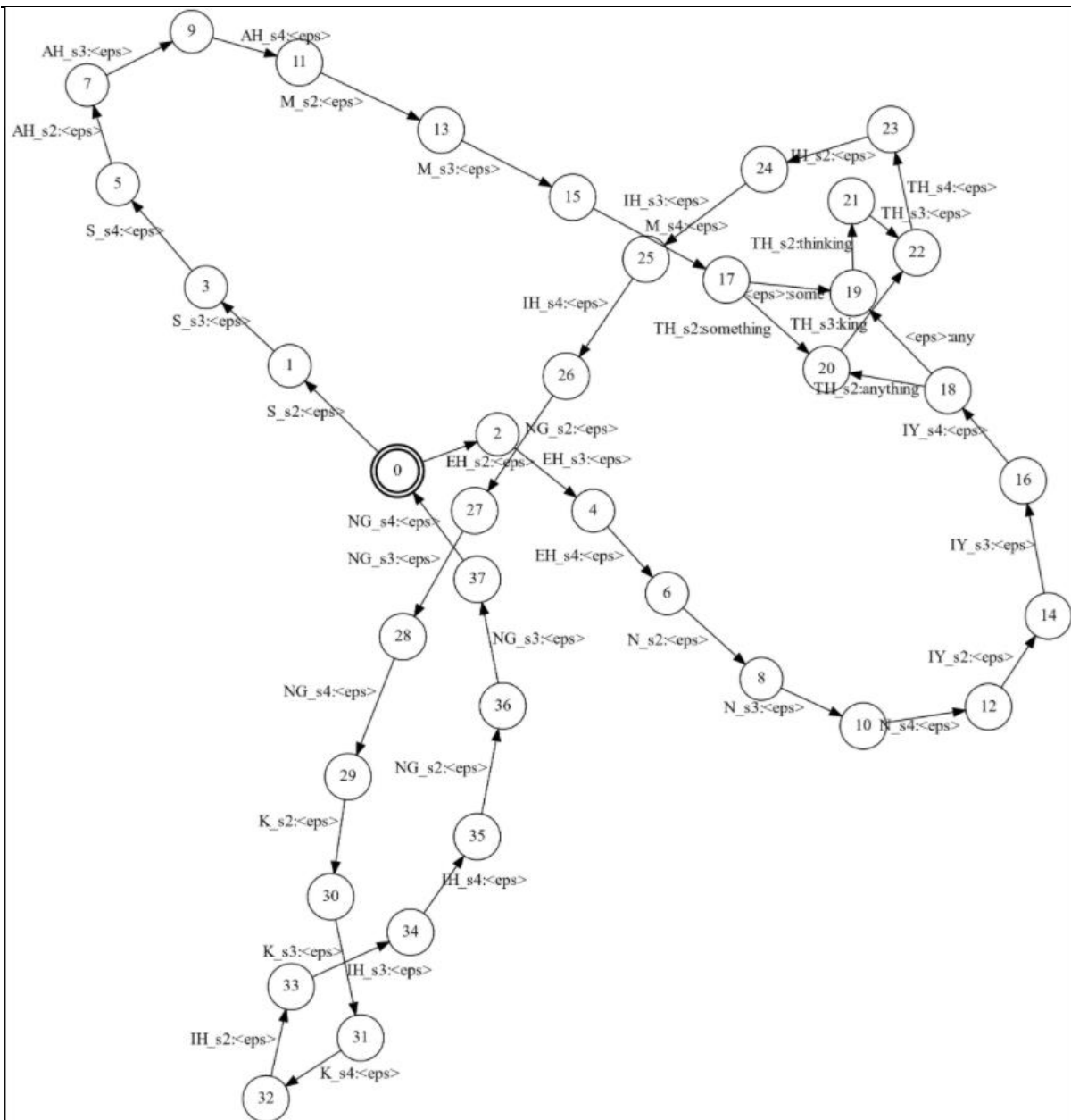
Slika 26. HCLG graf
