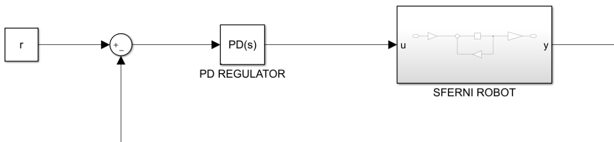
Slika 4.1. Shema zatvorenog kruga s PD regulatorom
