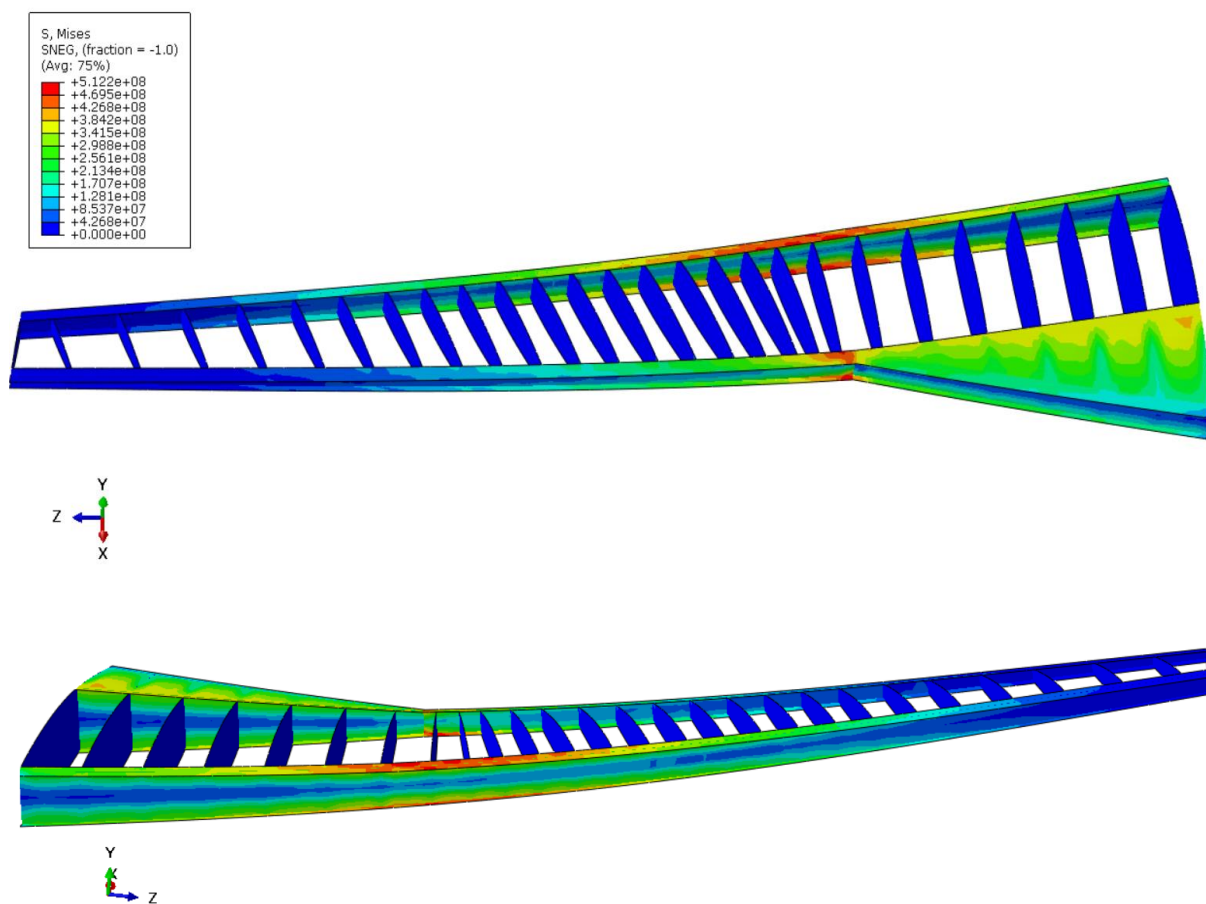
Slika 20. Raspodjela naprezanja [Pa] prema von Mises-u za model s kutom strijele 15°
