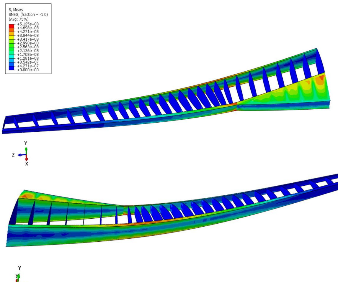
Slika 21. Raspodjela naprezanja [Pa] prema von Mises-u za model s kutom strijele krila 25^\circ
