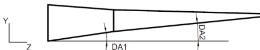
Slika 6. Parametri modela krila – bokocrt [6]
