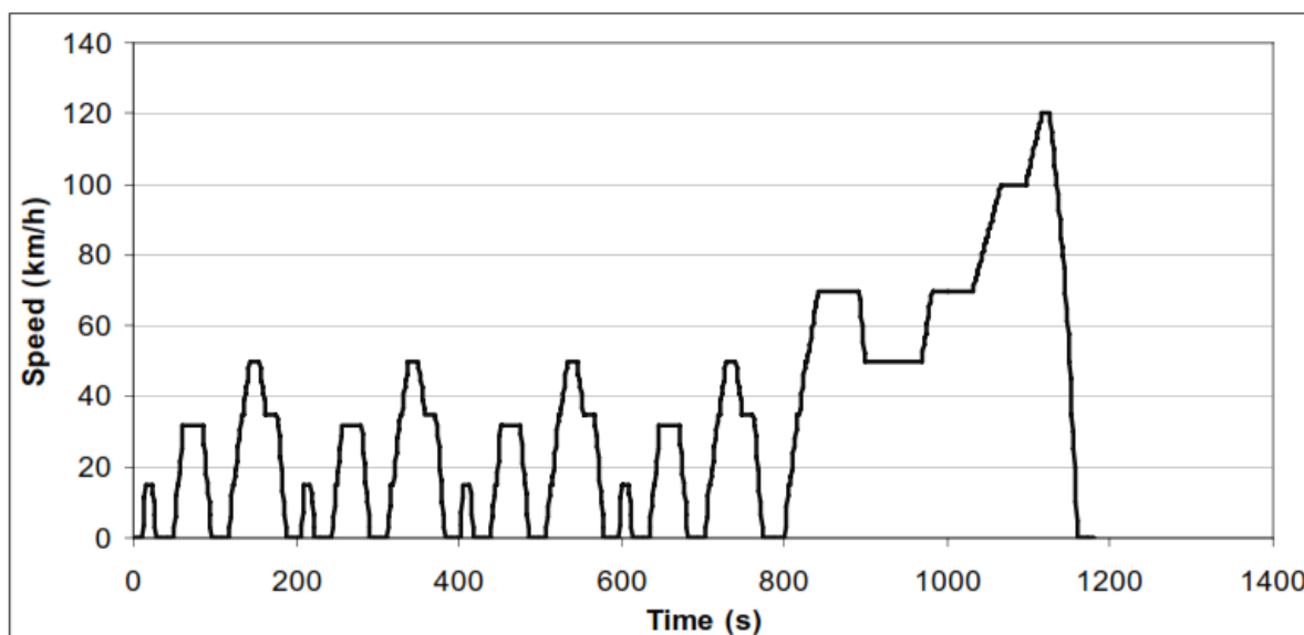
Slika 11. NEDC vozni ciklus [10]
