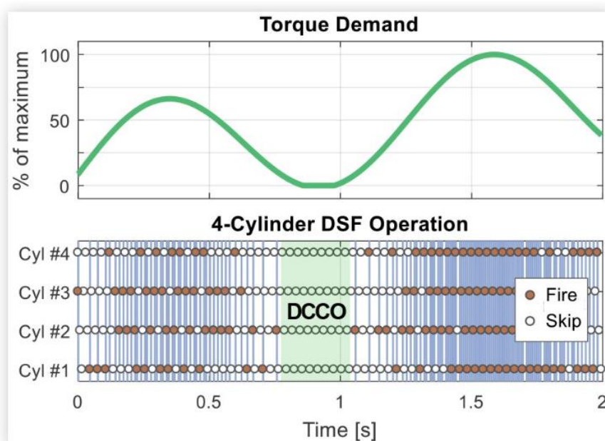
Slika 8. Primjer paljenja cilindara s DSF tehnologijom za 4-cilindrični motor [7]
