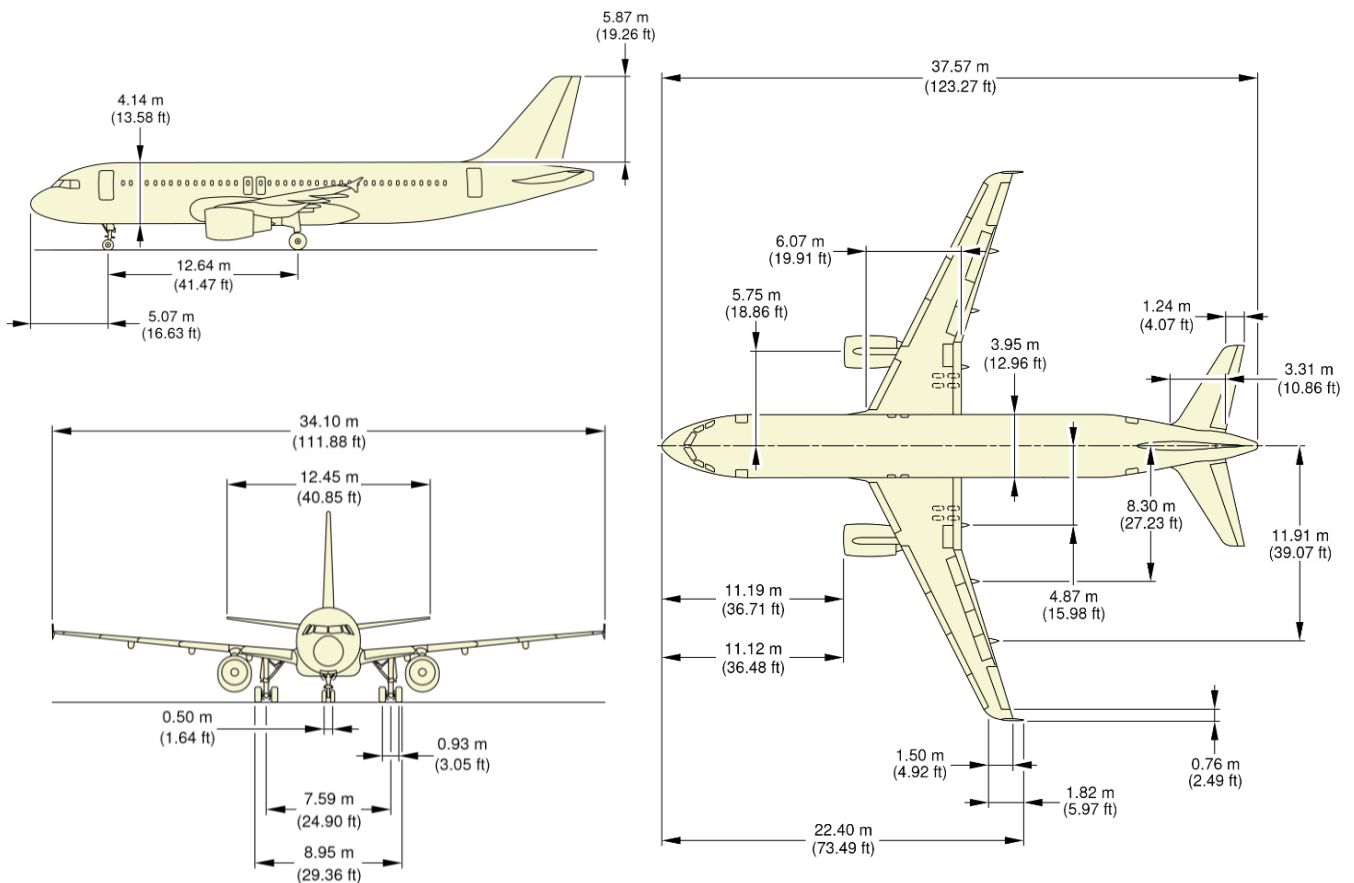
Slika 1.1: Airbus A-320 [1]
