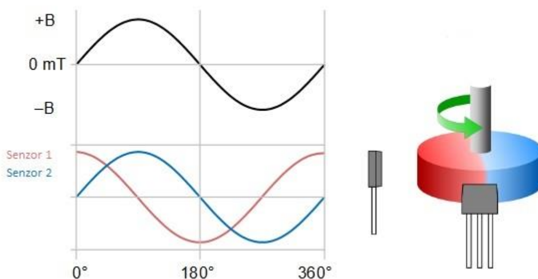
Slika 6. Izlazni signali linearnog Hallovog senzora [4]
