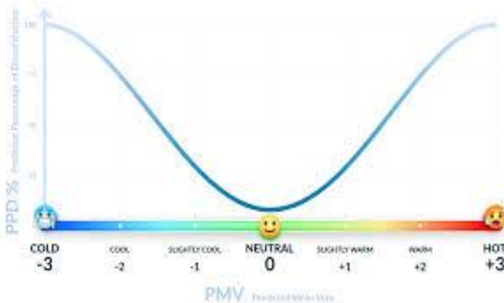
Slika 1 Prikaz predvidljivog postotka nezadovoljnih (PPD) u funkciji predvidljivog prosječnog vrednovanja (PMV)
