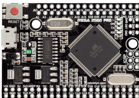
Slika 2.12 Arduino Mega 2560 PRO pločica [14]
