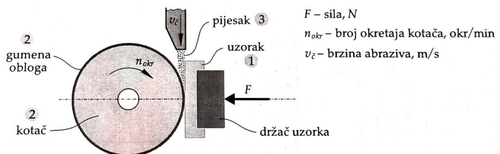
Slika 25 Skica uređaja "suhi pijesak/gumeni kotač" [18]
