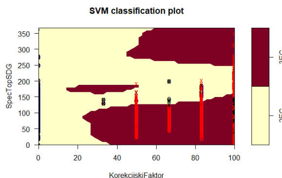
Slika 3-66 Klasifikacija strojem potpornih vektora ovisnosti potrošnje o modelu obračuna energije i korekcijskom faktoru.
