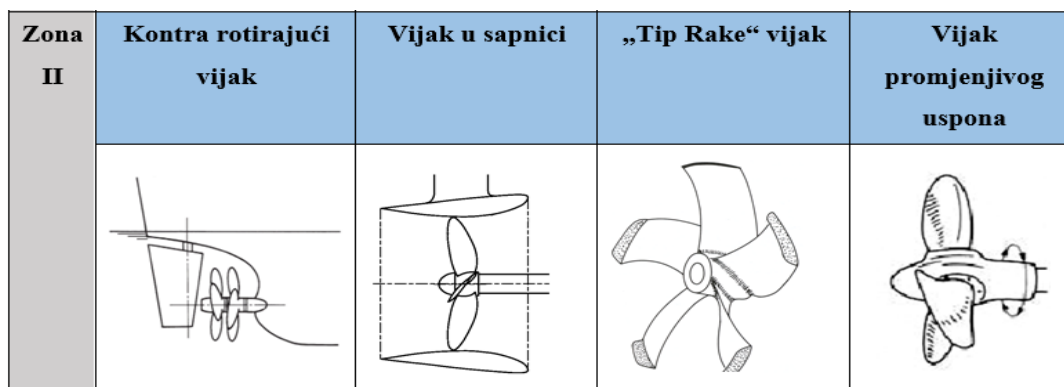
Slika 6. Glavni uređaji za uštedu energije
