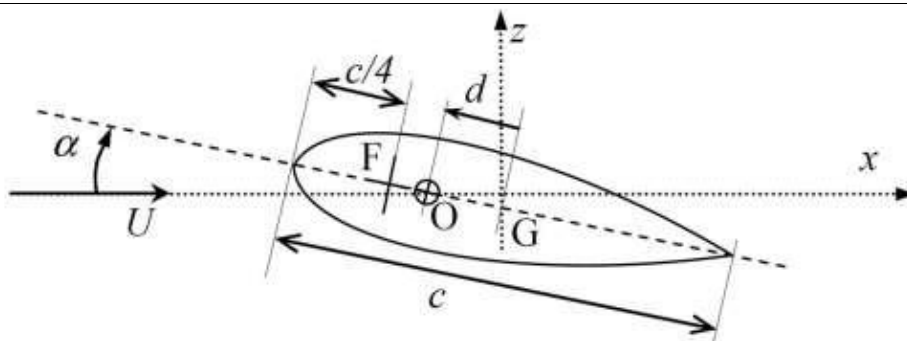
Slika 11. Strujni profil modela lepršanja [16]
