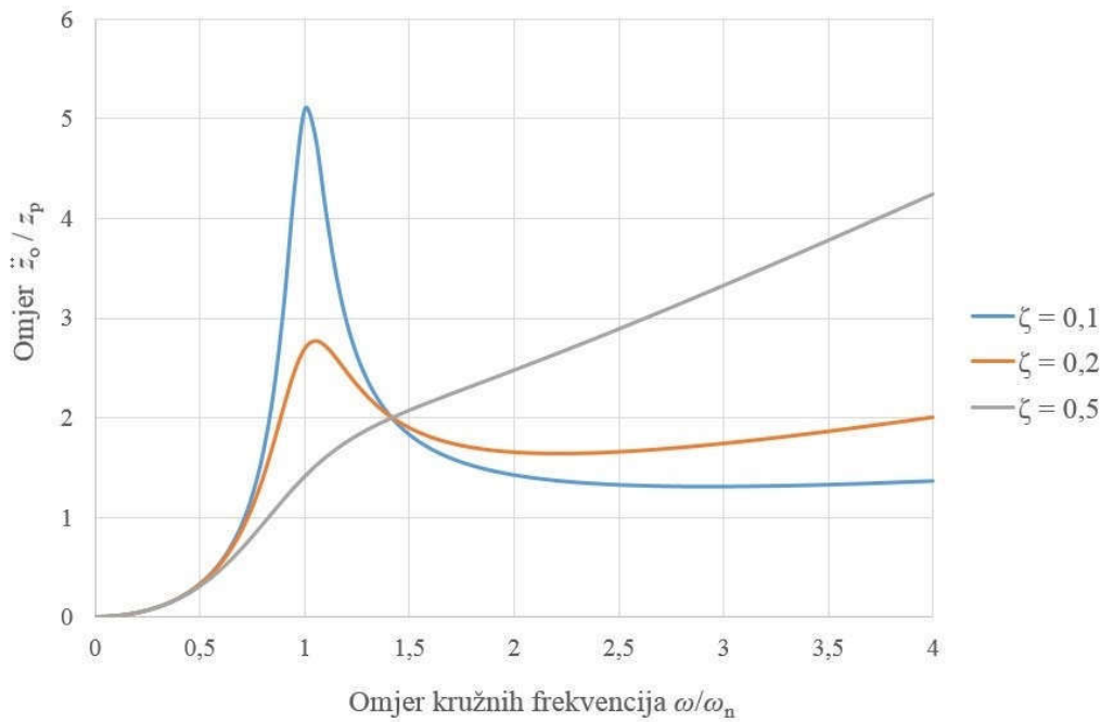
Slika 15. Dijagram ovisnosti omjera amplitude vertikalne akceleracije i pomaka o omjeru uzbudne i vlastite kružne frekvencije [7]
