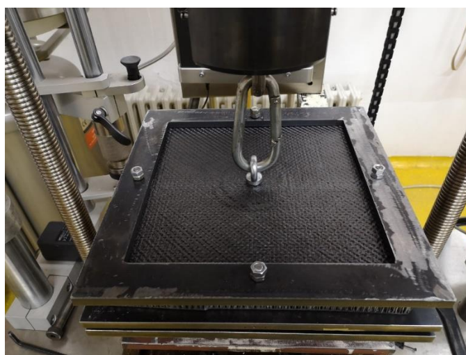
Slika 24. Prikaz testnog postava za ispitivanje prihvata sigurnosnih pojaseva [6]
