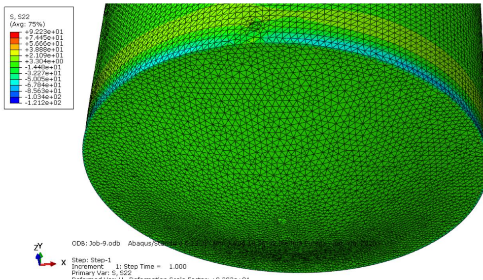
Slika 51. Raspored radijalnih naprezanja spremnika
