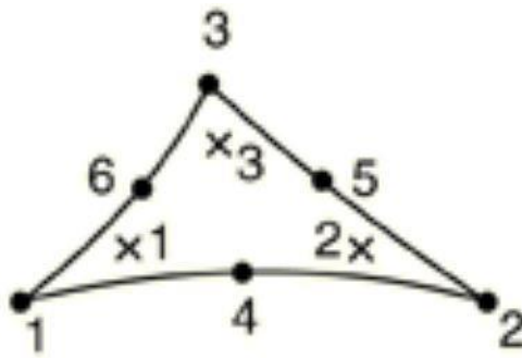
Slika 26. Ljuskasti trokutni element drugog reda [11]
