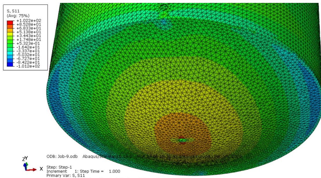
Slika 52. Raspodjela cirkularnih naprezanja spremnika
