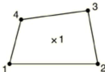
Slika 24. Ljuskasti četverokutni element prvog reda s reduciranom integracijom [11]
