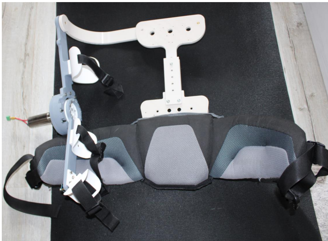
Slika 75. Cijeli sklop konstrukcije, prednji pogled
