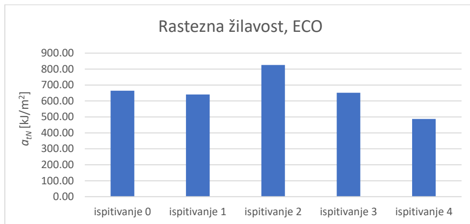
Slika 7.44. Usporedba vrijednosti rastezne žilavosti folije oznake ECO
