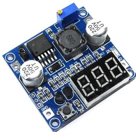
Slika 27. Modul za spuštanje napona LM2596-2 [18]
