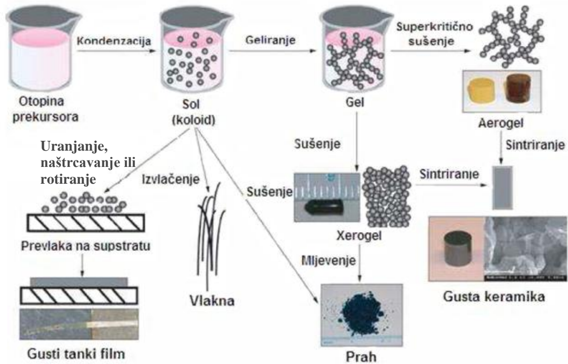
Slika 2. Priprema niskotemperaturne keramike sol-gel postupkom, dobivanje različitih proizvoda uz isti prekursor [2].
