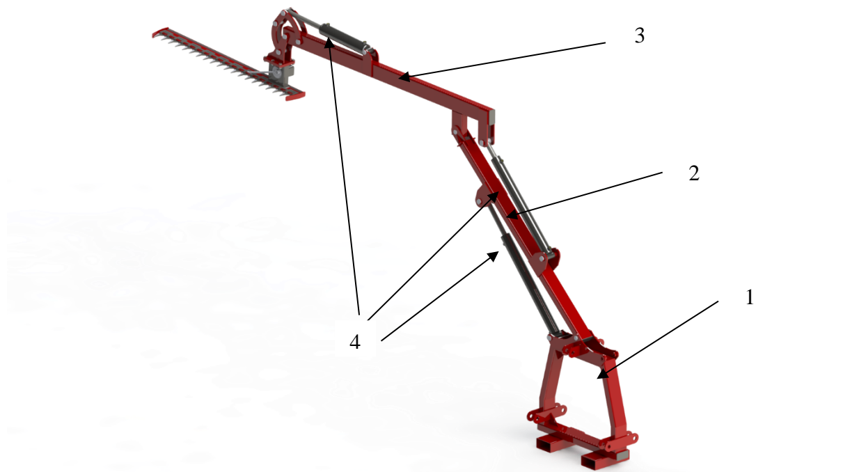
Slika 38. Mogući radni položaj sjekača
