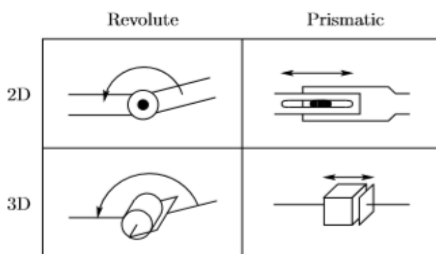
Slika 2 Rotacijski i translacijski zglob kinematičkog lanca [1]
