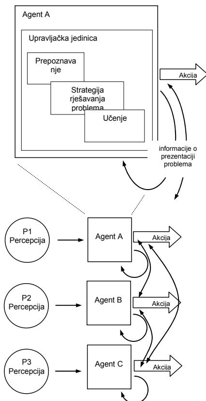
Slika 3-28. Struktura općenitog višegentskog sustava.
