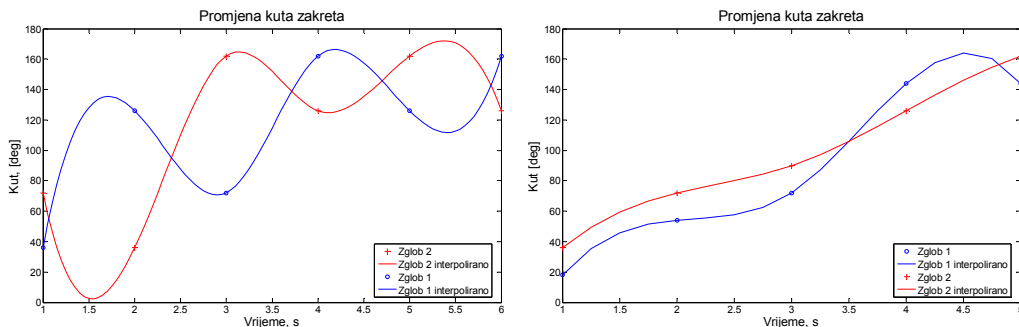
Slika 3-8. Ovisnost kuta zakreta o vremenu za dva slučaja konvergenције.
