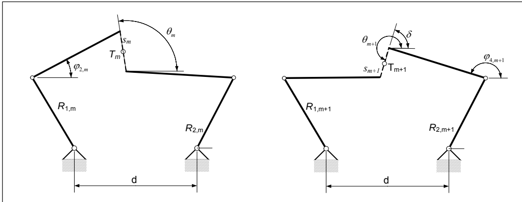
Slika 3-54. Rotacija spojnice s oko težišta T .
