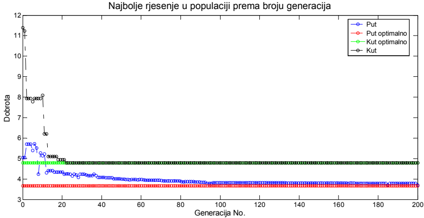
Slika 3-17. Konvergencija EA, slučaj II.
