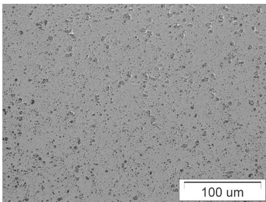
Slika 20. Fotografija poprečno prerezane površine uzorka dobivenog sljedećim režimom toplinske obrade: 450°C – ½ sata.
