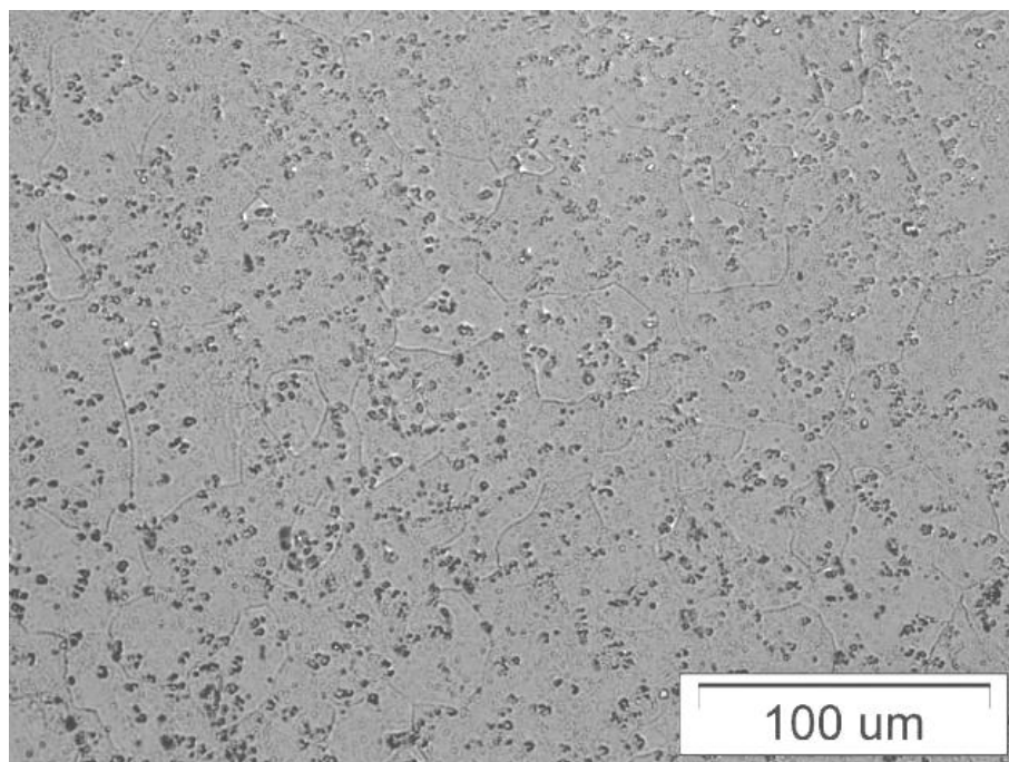
Slika 19. Fotografija bazne površine uzorka dobivenog sljedećim režimom toplinske obrade: 450°C – ½ sata.
