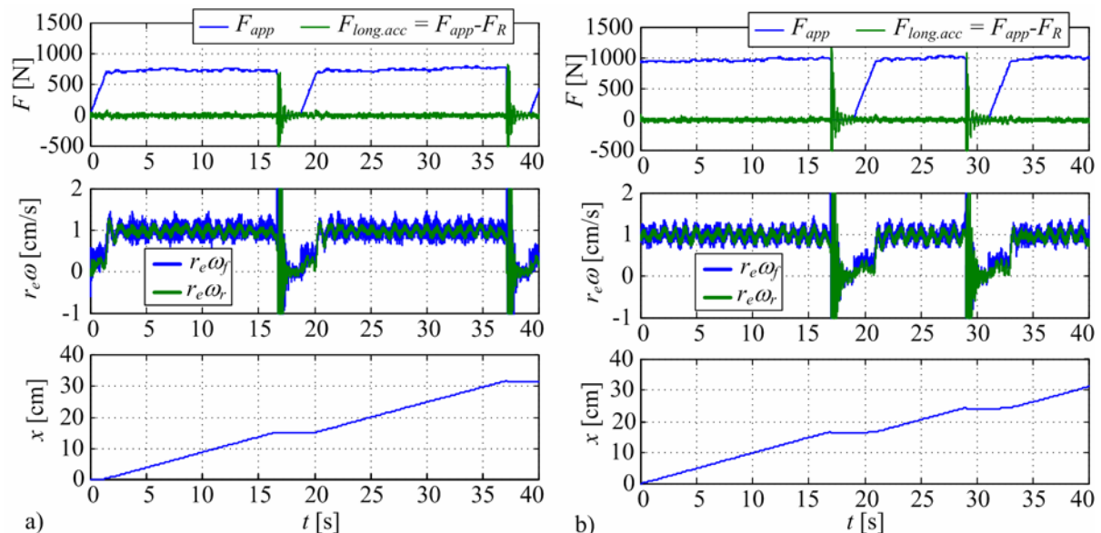
Slika 6-13. Analiza utjecaja sile otpora na ponašanje predloženog sustava regulacije vuče: a) F_R = 750 \text{ N} (20% više od STFP) i b) F_R = 950 \text{ N} (50 % više od STFP) ( varijanta 2 , \tau_{dwell} = 2 \text{ s} , v = 1 \text{ cm/s} ).
