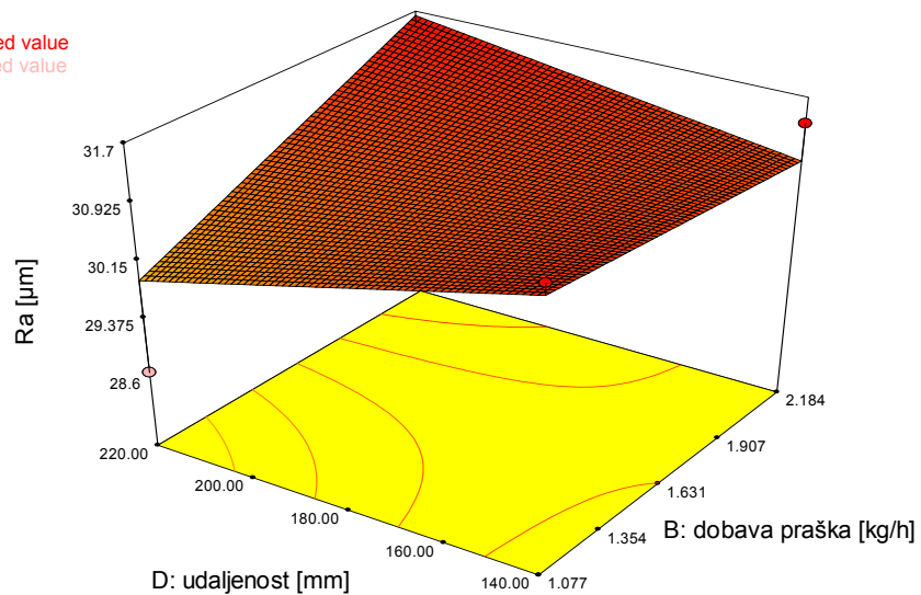
Slika 4.39 3D prikaz matematičkog modela ovisnosti parametra hrapavosti R_a naštrecanog sloja o ulaznim parametrima procesa plinskog naštrecavanja (konstantni su: A = 10 m/min, C = 6 mm, E = 2 bar).
