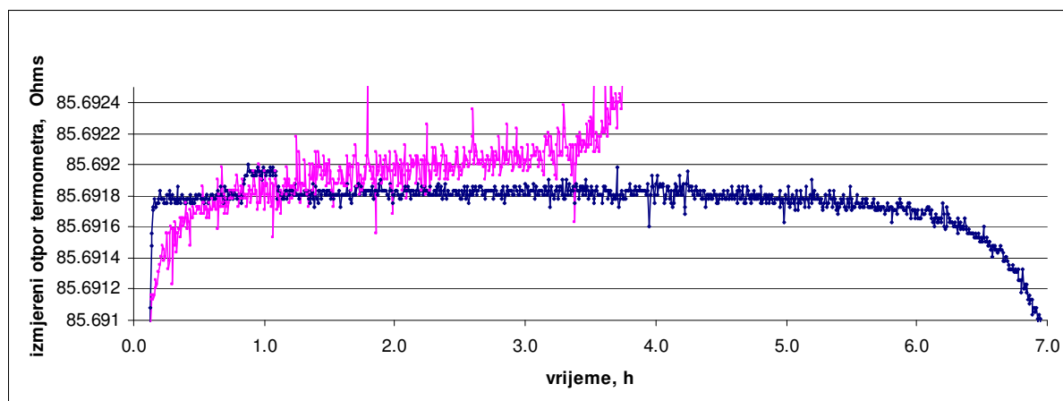
Slika 53 Rezultati usporedbe temperature taljenja i skrućivanja fiksne točke aluminija za procjenu standardne nesigurnosti ispravka C_{xt/1}
