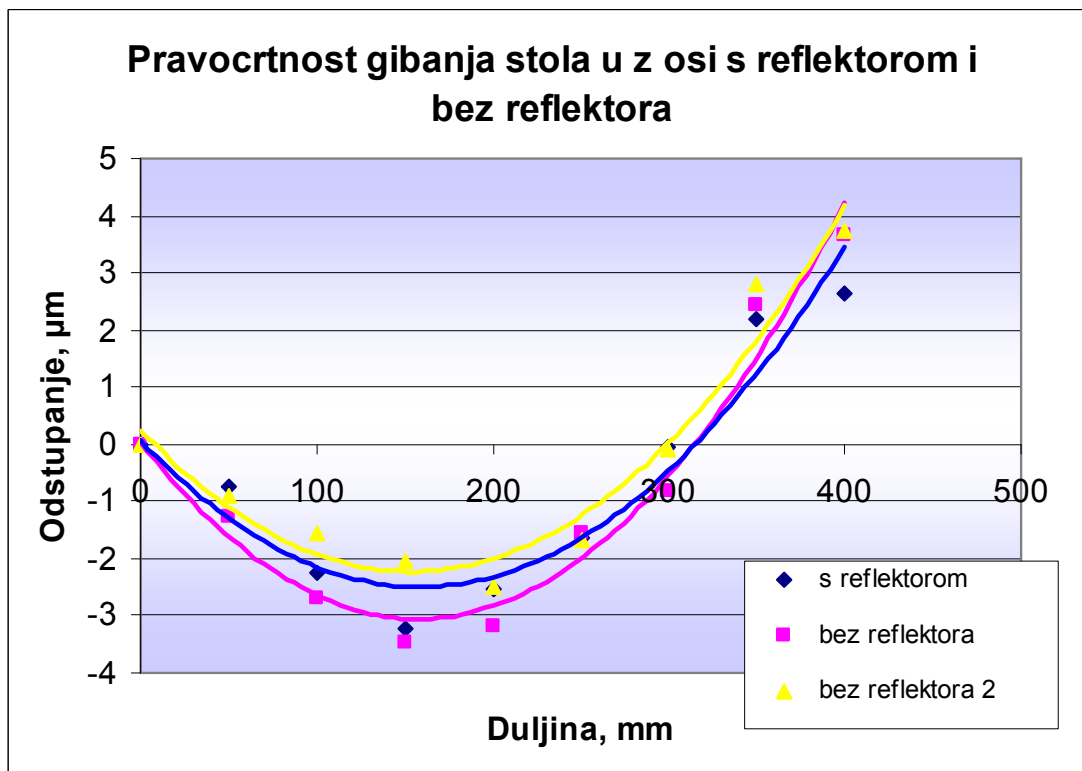
Slika 114. Pravocrtnost gibanja stola u z osi
