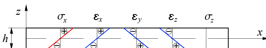
Slika 73. Točna raspodjela komponenata napreznanja i deformacija za čisto savijanje ploče
