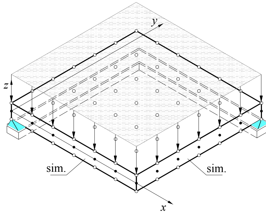
Slika 95. Izometrijski prikaz četvrtine kvadratne ploče slobodno oslonjena po svim stranicama
