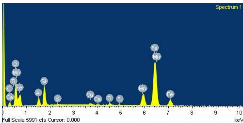
b) Dobiveni spektar analize pozicije Spectrum1 u metalu zavara na uzorku B1
