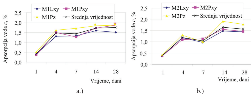
Slika 8.27. Apsorpcija vode kod miješanog materijala: a.) rastezna ispitna tijela, b.) savojna ispitna tijela
