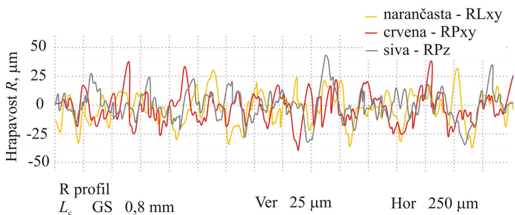
Slika 8.40. Hrapavost površine ispitnih tijela načinjenih od recikliranog materijala
