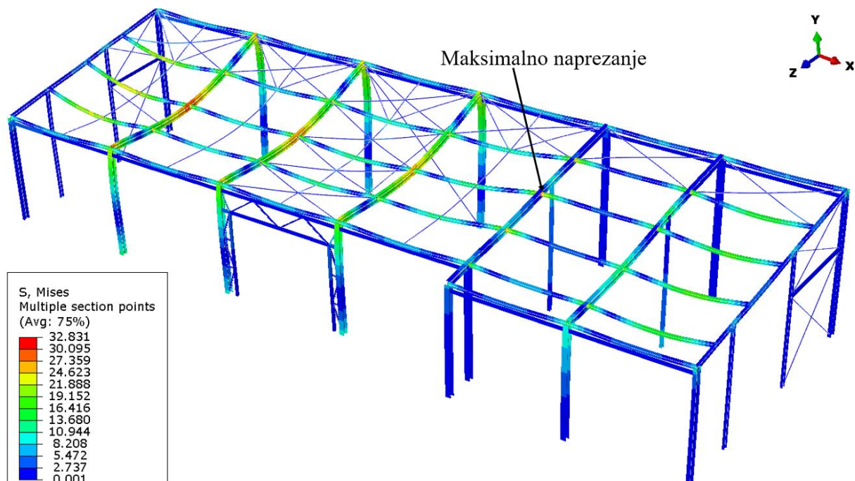
Slika 4.12. Raspodjela ekvivalentnih naprežanja u nosivoj konstrukciji, u \text{N/mm}^2 , uslijed opterećenja od vlastite težine i težine instalacija
