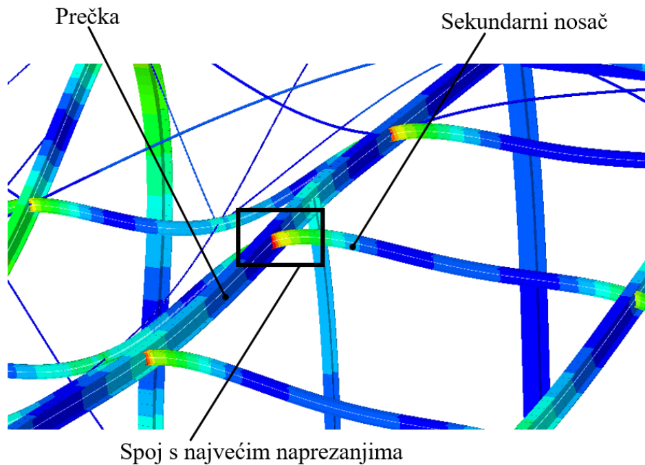
Slika 4.27. Prikaz spoja s najvećim ekvivalentnim naprezanjima po von Misesu u N/mm^2
