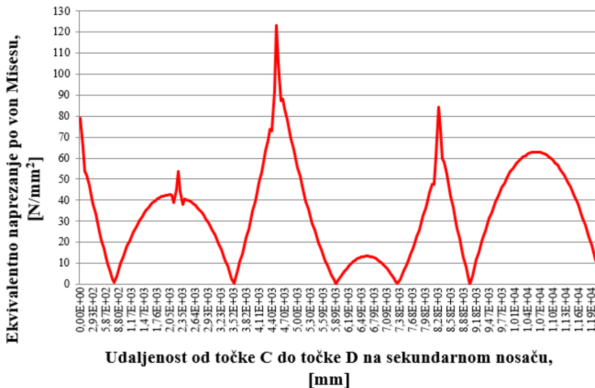
Slika 4.28. Dijagram ekvivalentnog naprezanja po von Misesu u N/mm^2
