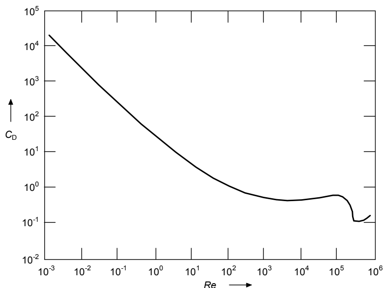
Slika 2-15. Dijagramski prikaz ovisnosti faktora otpora trenja C_D o Reynoldsovoj značajci za pojedinačno nestrujanu kuglu
