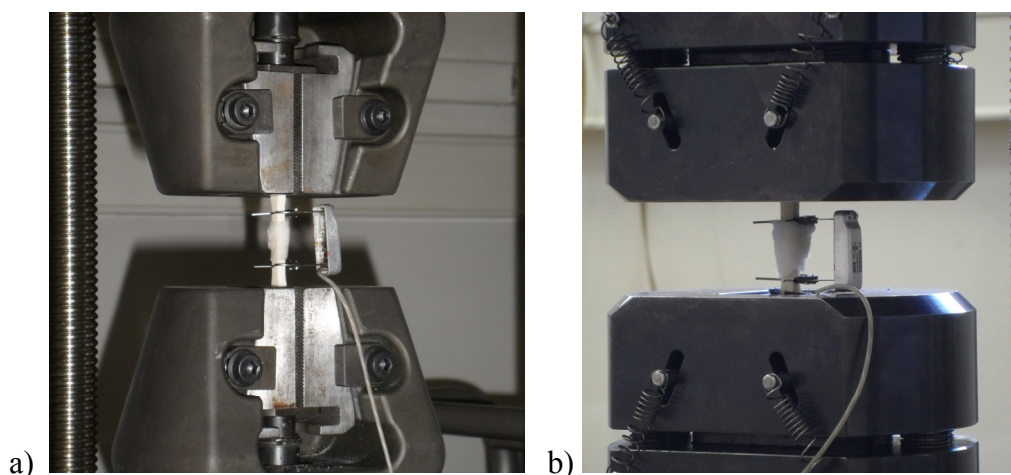
Slika 30. Uzorak govedeg kortikalnog koštanog tkiva omotan vlažnom vatom tijekom a) vlačnog i b) tlačnog eksperimenta
