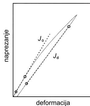
Slika 40. Shematski prikaz ovisnosti napreznjenja o deformaciji za određivanje podatljivosti pri rasterećenju ( J_d ) i početne podatljivosti ( J_0 ) [105]
