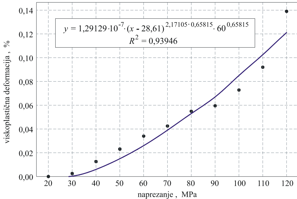
Slika 55. Ovisnost viskoplastične deformacije o naprežanju za slučaj puzanja za govede kortikalno koštano tkivo
