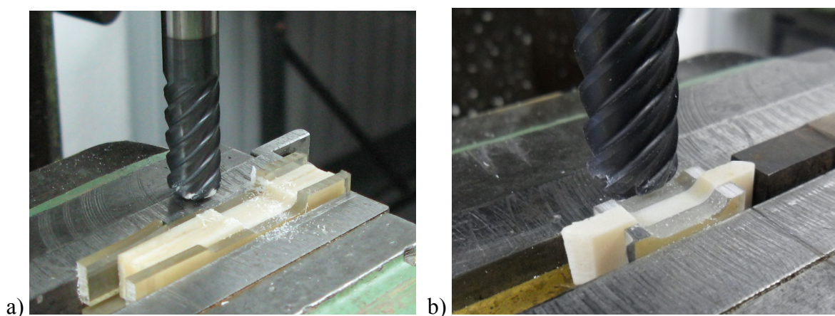
Slika 28. Obrada epruvete dimenzija a) 10(6) \times 3 mm u longitudinalnom smjeru, b) 8(4,5) \times 3 mm u tranverzalnog smjeru glodalom 308.120.25
