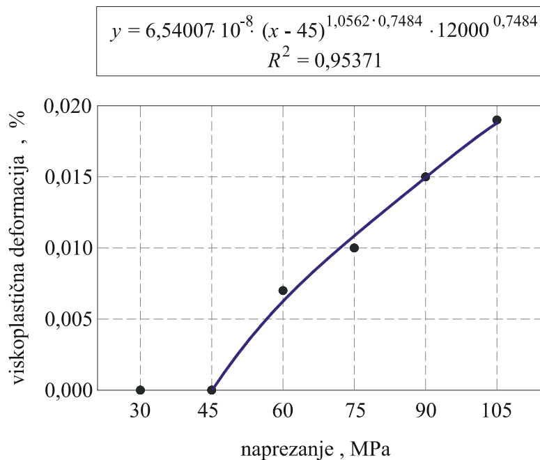
Slika 63. Ovisnost viskoplastične deformacije o naprezanju za ljudsko kortikalno koštano tkivo
