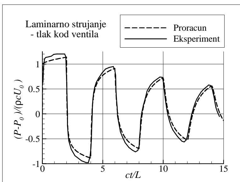
Sl. 4.11 Proračunati i izmjereni [58] tijek promjene tlaka kod ventila
