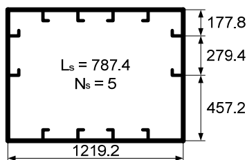
Slika 4.2 Dimenzije modela P1.
