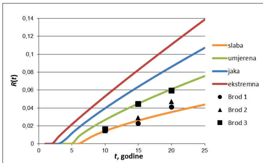
Slika 2.13 - Gubitak momenta otpora poprečnog presjeka za različite oštine korozije prema ABS-u
