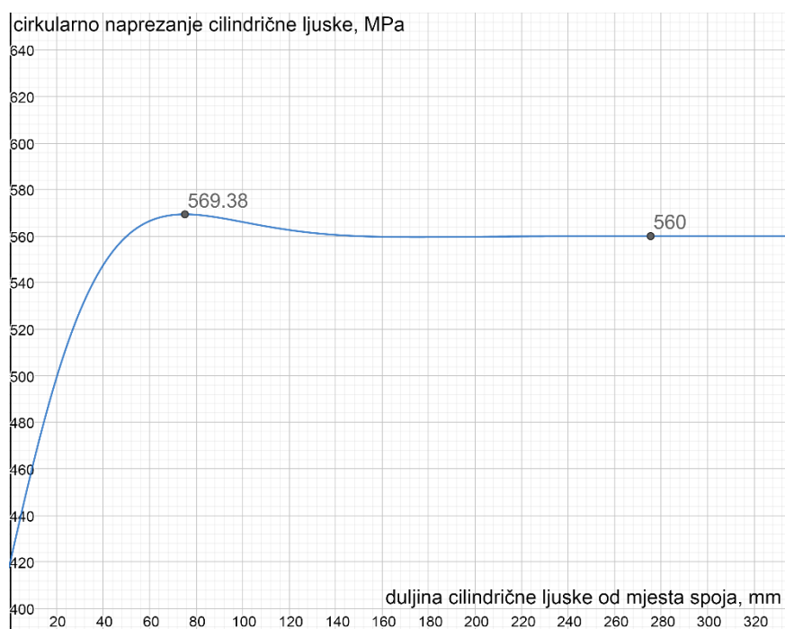
Slika 34. Raspodjela cirkularnog naprezanja duž izvodnice cilindrične ljsuske
