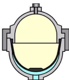
Slika 2. Membranski akumulator
