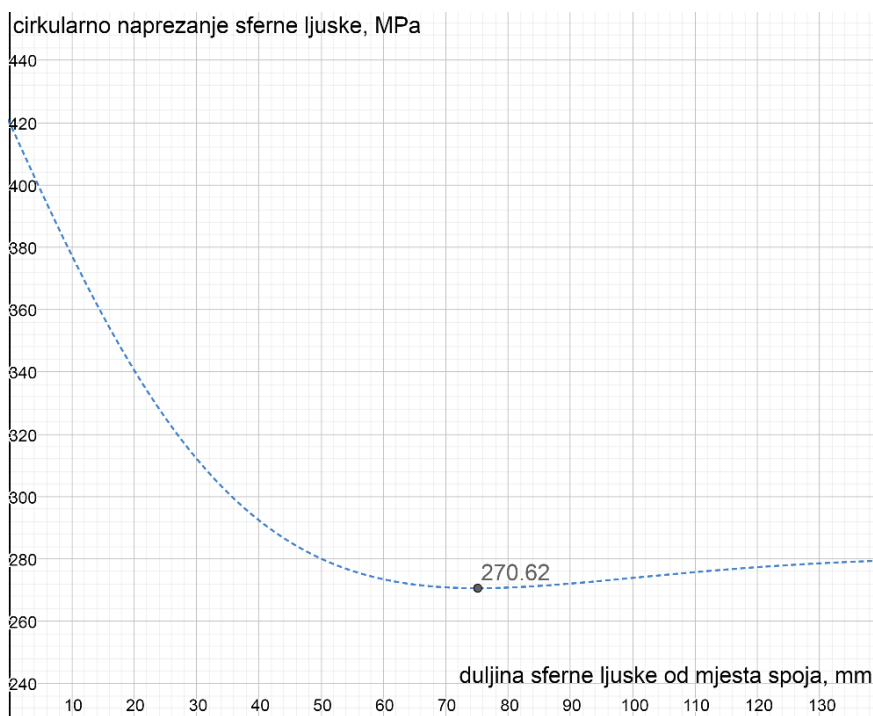
Slika 35. Raspodjela cirkularnog naprezanja duž izvodnice sferne ljsuske
