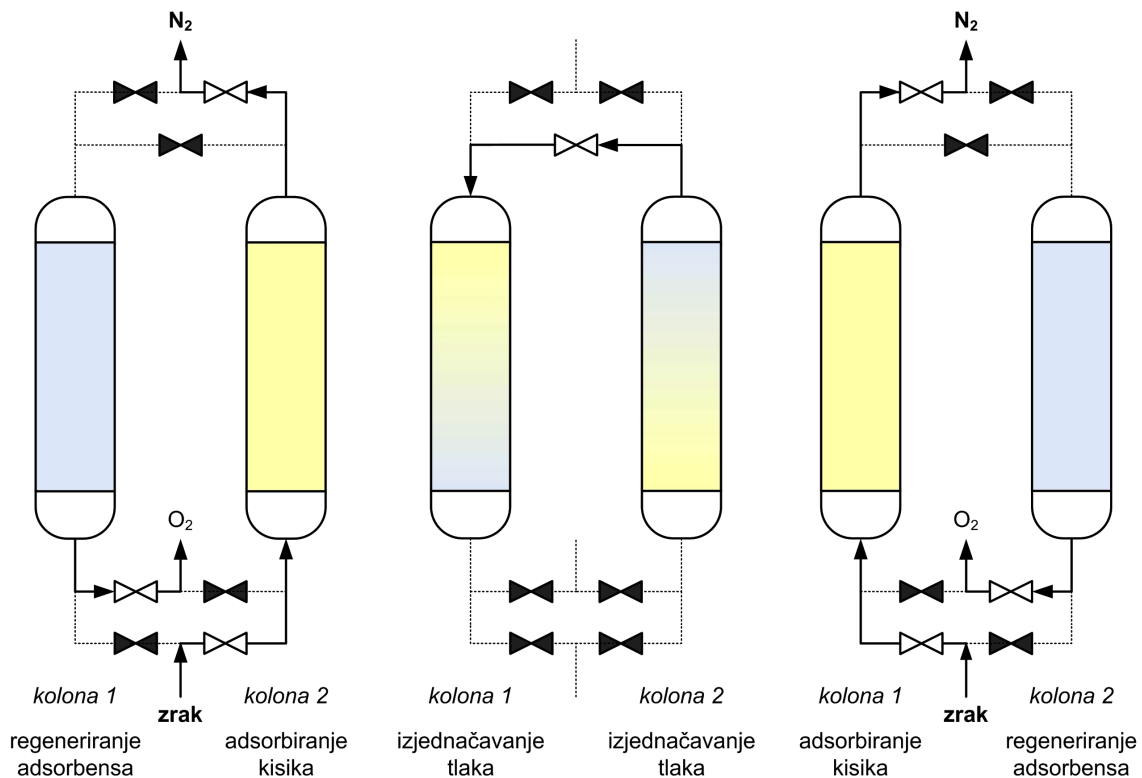
SI. 2.10. PSA postupak dobivanja dušika
