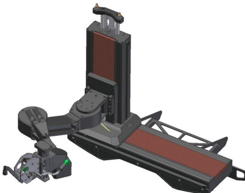
Slika 11. Manipulator Prima [18]
