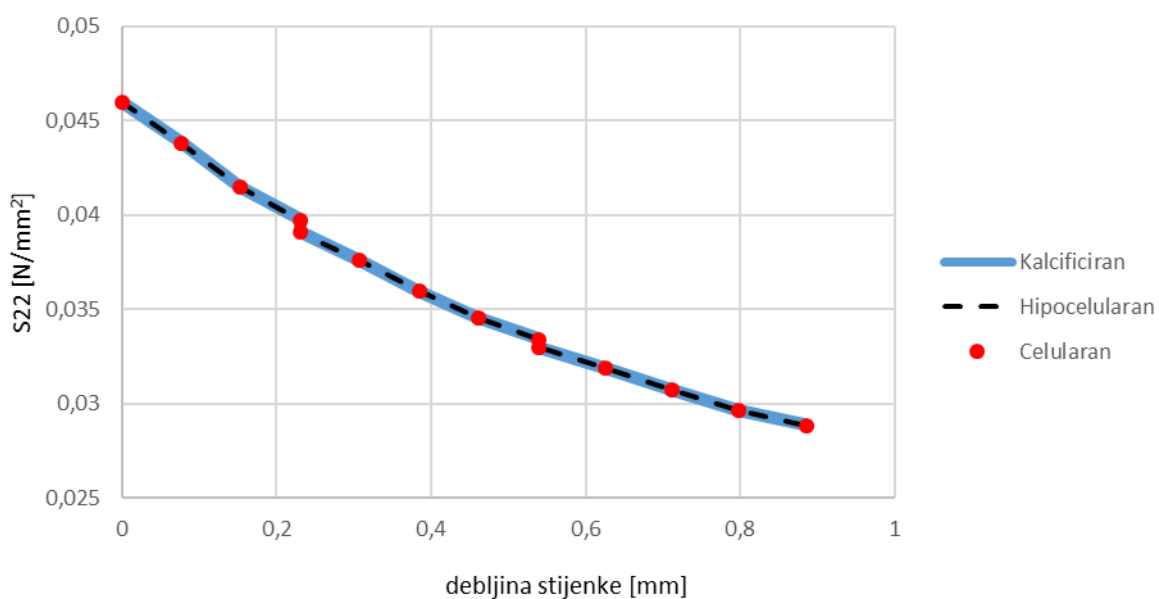
Slika 44. Cirkularno naprezanje \sigma_{22} [N/mm 2 ] po debljini stijenke
