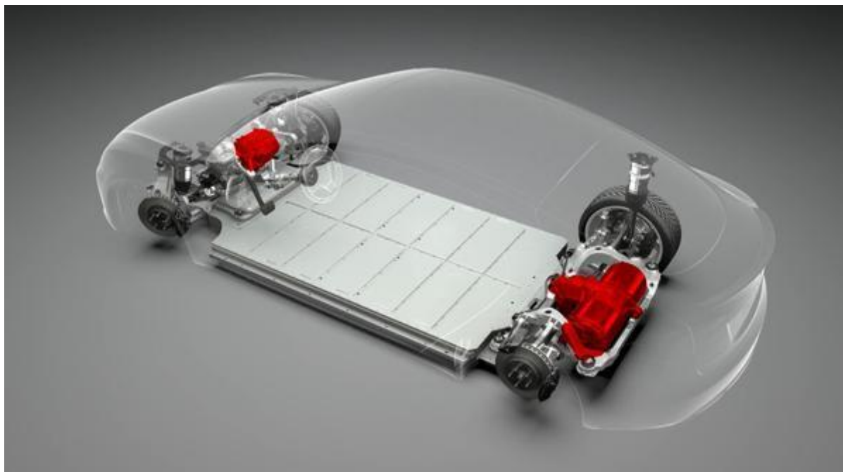
Slika 28 „Floor“ konfiguracija baterijskog paketa (Tesla Model S)
