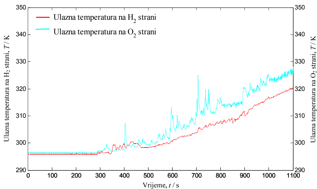
Slika 7.7 Promjena ulazne temperature na vodikovoj, odnosno kisikovoj strani (isključenje pumpi nakon 300 s)
