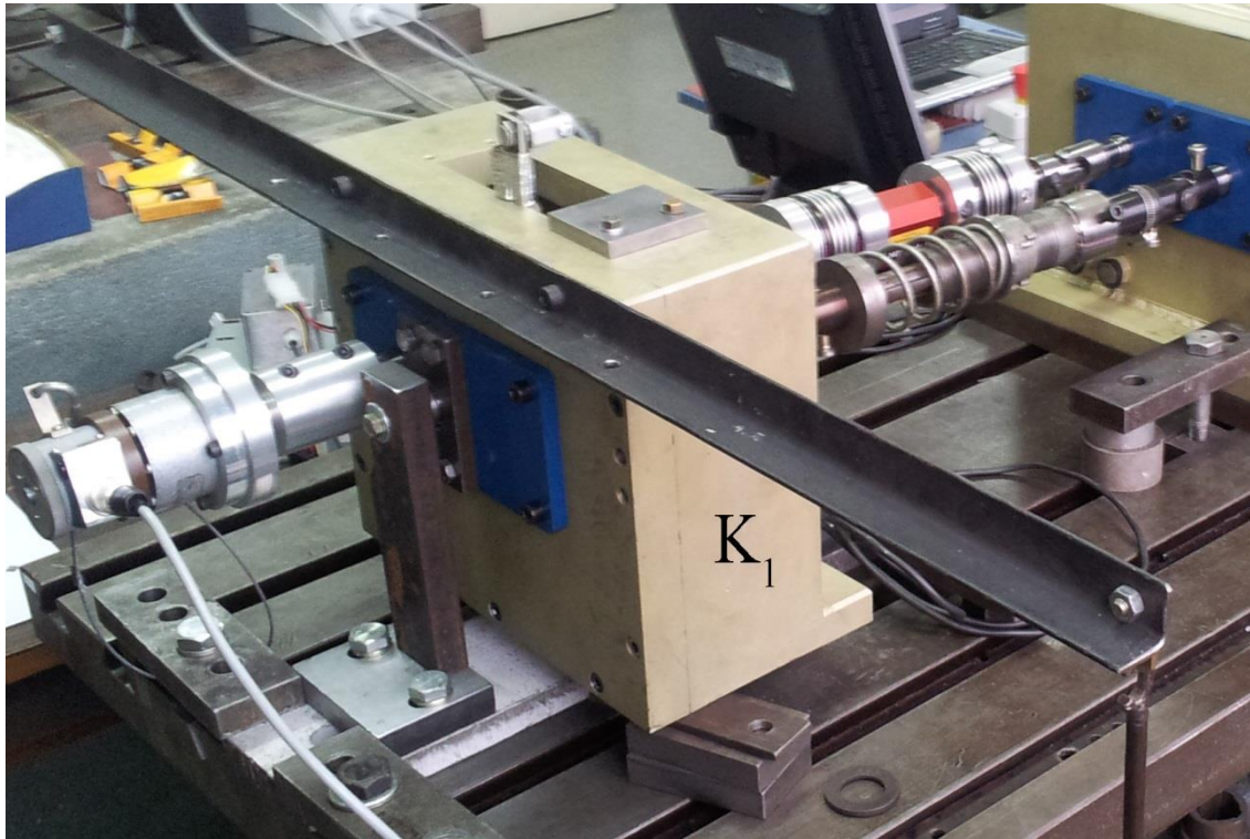
Slika 4.7 Ispitni prijenosnik
