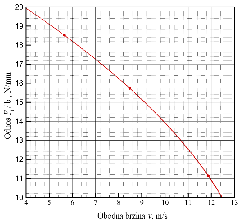
Slika 5.55 Ovisnost odnosa obodne sile i širine zupčanika od PA 6 kod različitim obodnim brzinama
