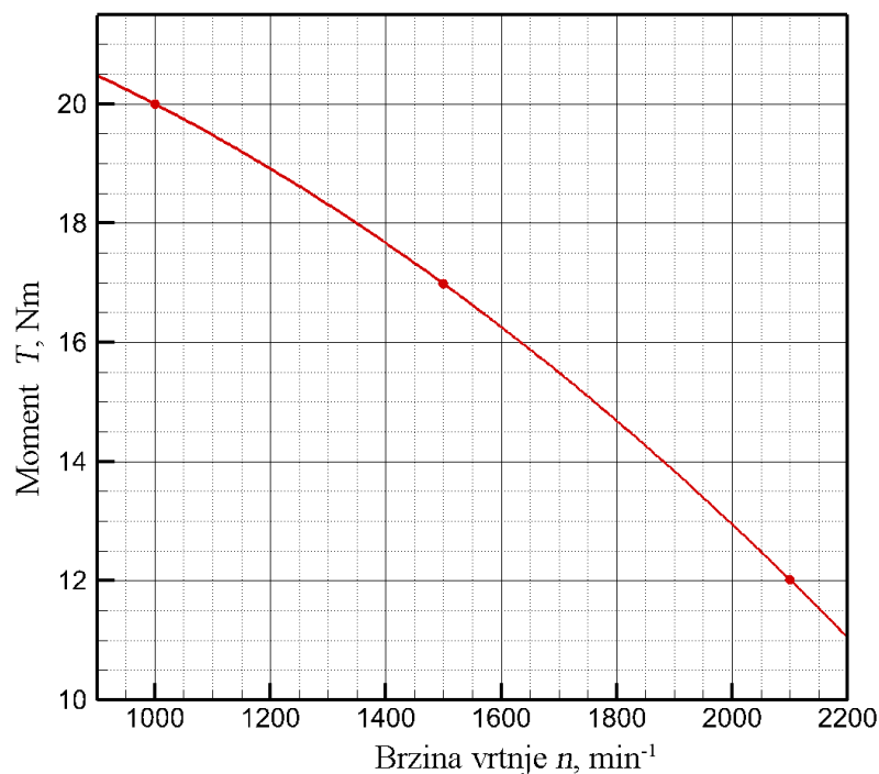
Slika 5.54 Opteretivost zupčanika od PA 6 kod različitim brzinama vrtnje
