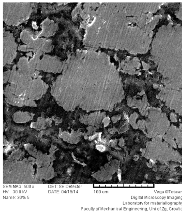
Slika 49. Detalj površina uzorka Ti30Mg nakon korozivskog ispitivanja [225]
