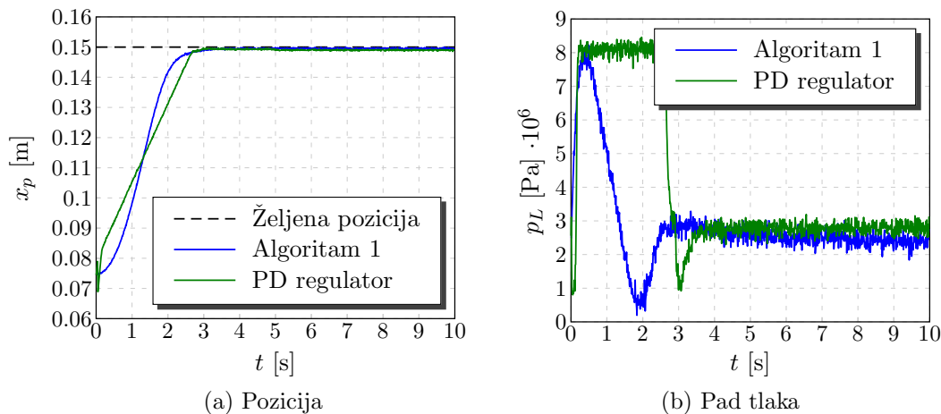
Slika 6.23: Eksperimentalni rezultati upravljanja translacijskim gibanjem: varijable stanja u ovisnosti o vremenu.
