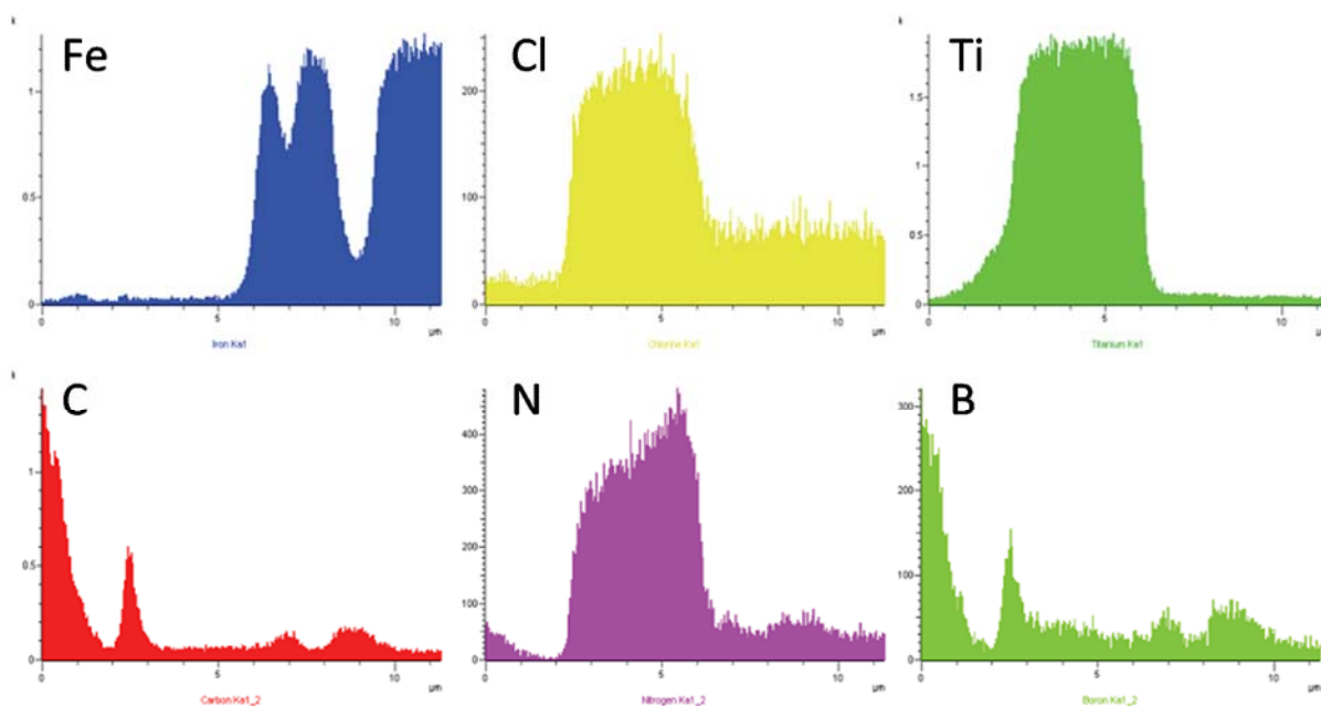
Slika 4.17 EDS linijska analiza poprečnog presjeka uzorka A3 s TiBN prevlakom na čeliku X38CrMoV5-3
