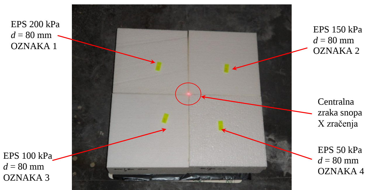
Sl.- 54. Postav ispitnih uzoraka na slikovnu ploču za pokus karakterizacije komponenata sustava očitavanja.
