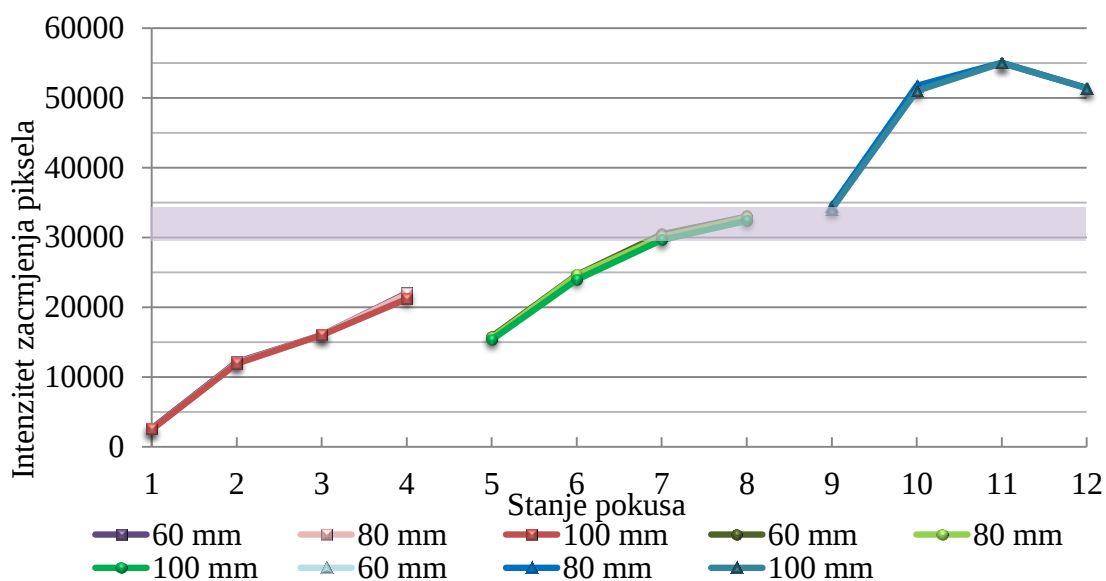
Sl.- 52. Grafički prikaz ovisnosti intenziteta zacrnjenja piksela o parametrima eksponiranja za stanja pokusa 1 - 12.
