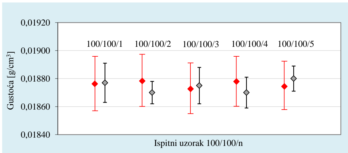
Sl.- 86. Usporedivost za razinu povjerenja od 95 % modelom određenih strukturnih gustoća, \rho_n , za pet eksponiranja i prividnih gustoća, \rho_{prividno} , dobivenih konvencionalnom metodom, za ispitne uzorke ekspandiranoga polistirena oznaka 100/100/n, gdje je n = 1 do 5.
